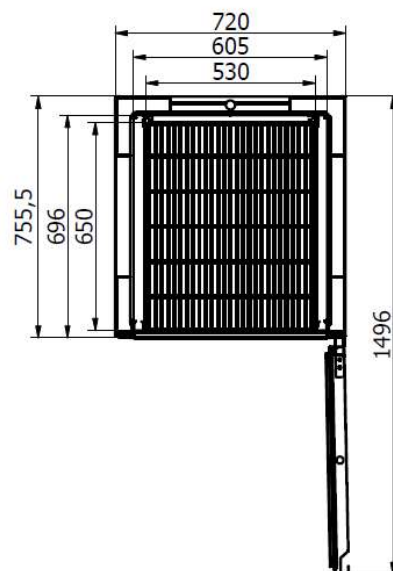
Vue de haut porte ouverte
